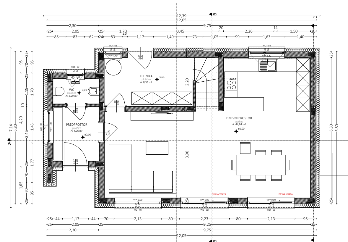
TLORIS PRITLIČJA
