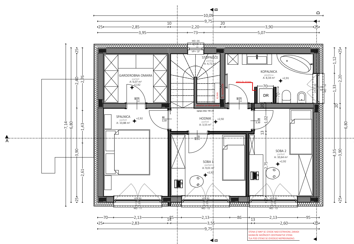
TLORIS MANSARDE
